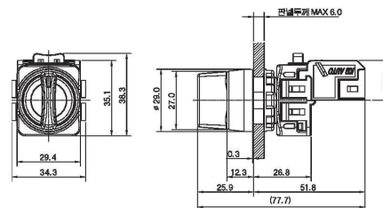
셀렉터 스위치 2단 (Selector s/w 2stage) (KGS - H2M1) M(MAIN-AUX), L(LIGHT)
