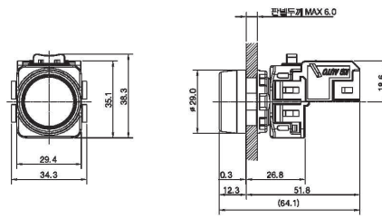
누름버튼 스위치 (Push button) (KGF - HM1G) - H(HORN)
